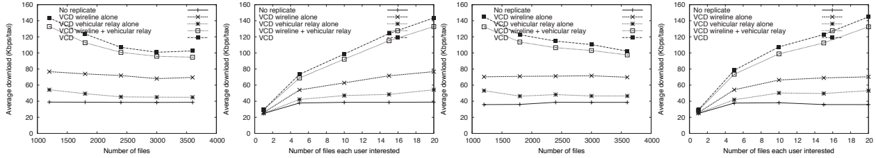
(a) Uniform: vary # f les (b) Uniform: vary # f les per user (c) Zipf-like: vary # f les (d) Zipf-like: vary # f les per user
